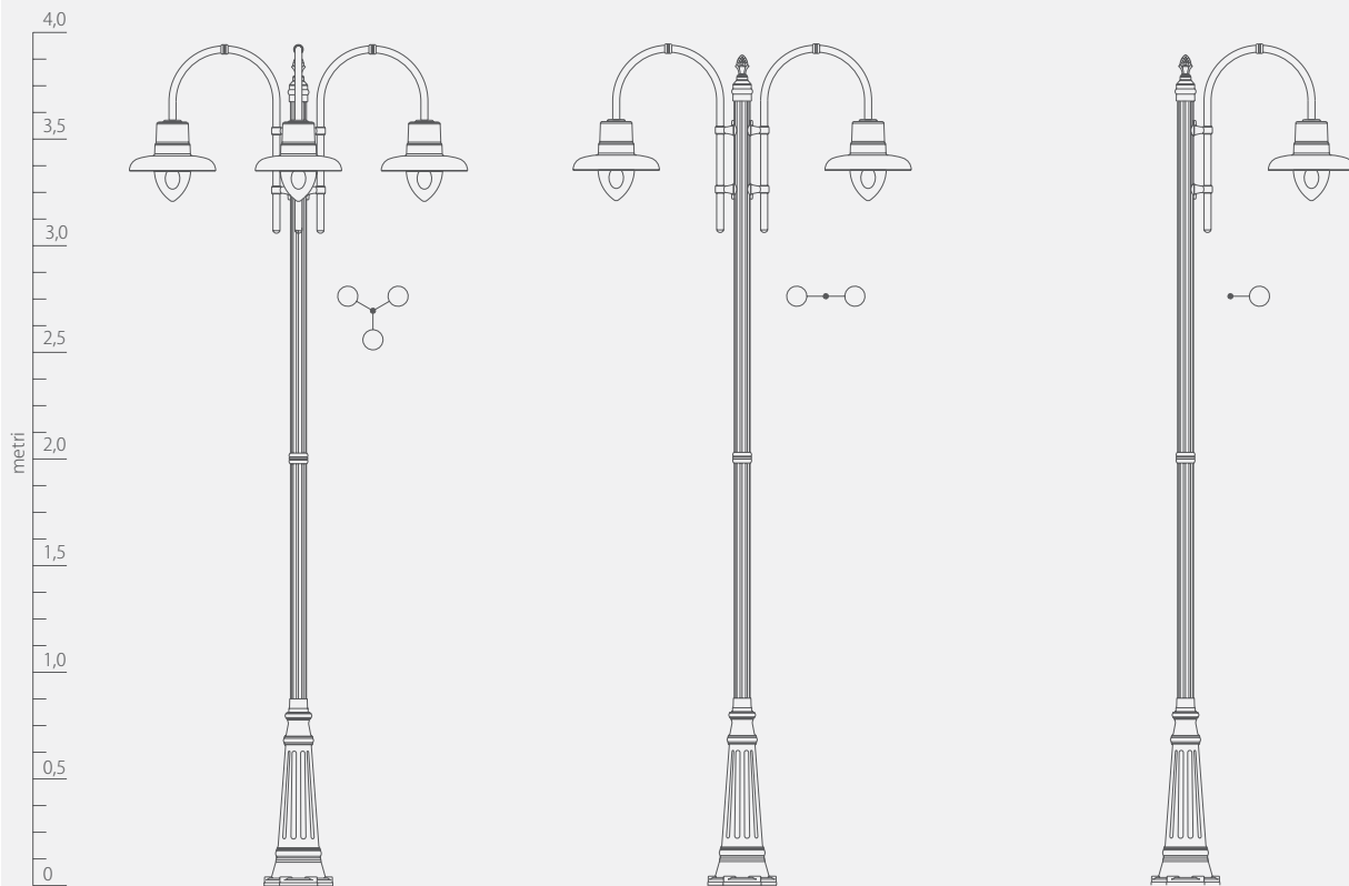
▶ modello: GEMMA CR articolo: 75.B8/3.44 altezza tot. cm 397 palo tipo: 75/B8
