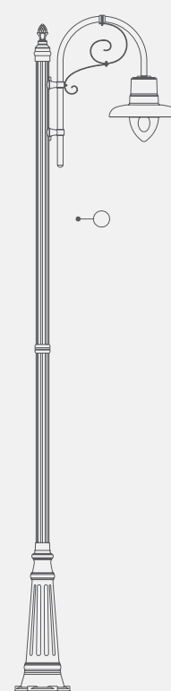
▀ modello: GEMMA CR articolo: 75.B8/1.445R altezza tot. cm 397 palo tipo: 75/B8
