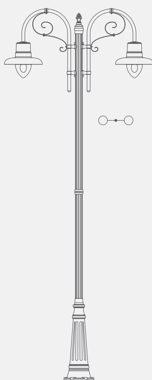
▀ modello: GEMMA CR articolo: 75.B8/2.445R altezza tot. cm 397 palo tipo: 75/B8
