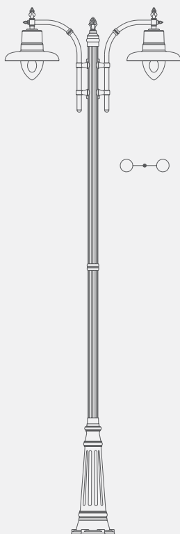
▀ modello: GEMMA CR articolo: 75.B8/2.90B altezza tot. cm 394 palo tipo: 75/B8
