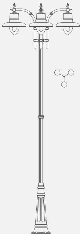
▀ modello: GEMMA CR articolo: 75.B8/3.90B altezza tot. cm 394 palo tipo: 75/B8
