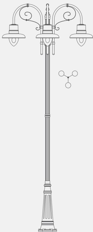
▀ modello: GEMMA CR articolo: 75.B8/3.445R altezza tot. cm 397 palo tipo: 75/B8
