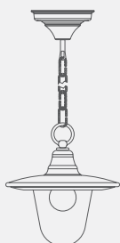
modello: AGENA articolo: 4S misure mm: L255 x H725
