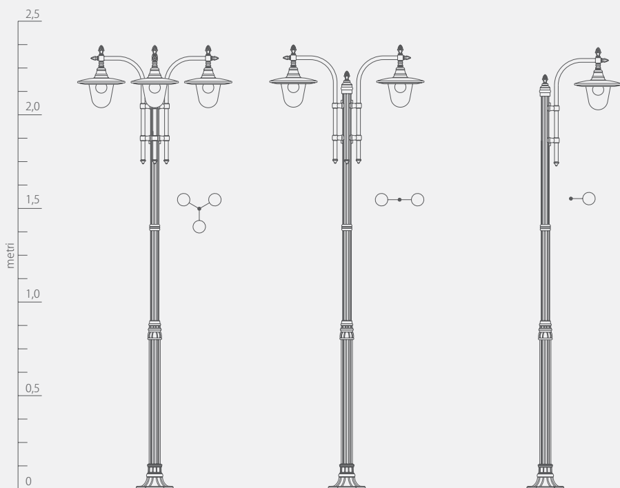
▸ modello: AGENA articolo: 60.45/90.3 altezza tot. cm 237 palo tipo: 60.45
