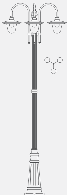
modello: AGENA articolo: 60.B5/3 altezza tot. cm 249 palo tipo: 60/B5
