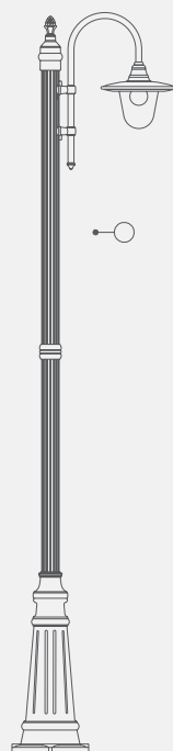
modello: AGENA articolo: 60.B5/1 altezza tot. cm 249 palo tipo: 60/B5
