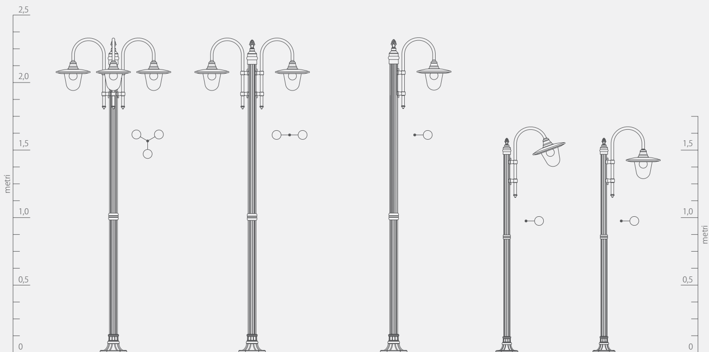
▸ modello: AGENA articolo: 60/3 altezza tot. cm 233 palo tipo: 60
