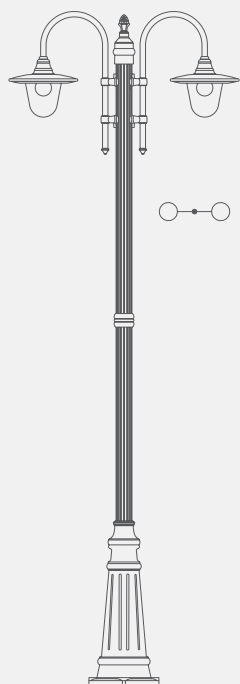
modello: AGENA articolo: 60.B5/2 altezza tot. cm 249 palo tipo: 60/B5
