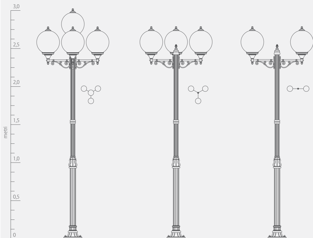
modello: ELIOS 300 articolo: 75.60/K4.4.P altezza tot. cm 297 palo tipo: 75.60
