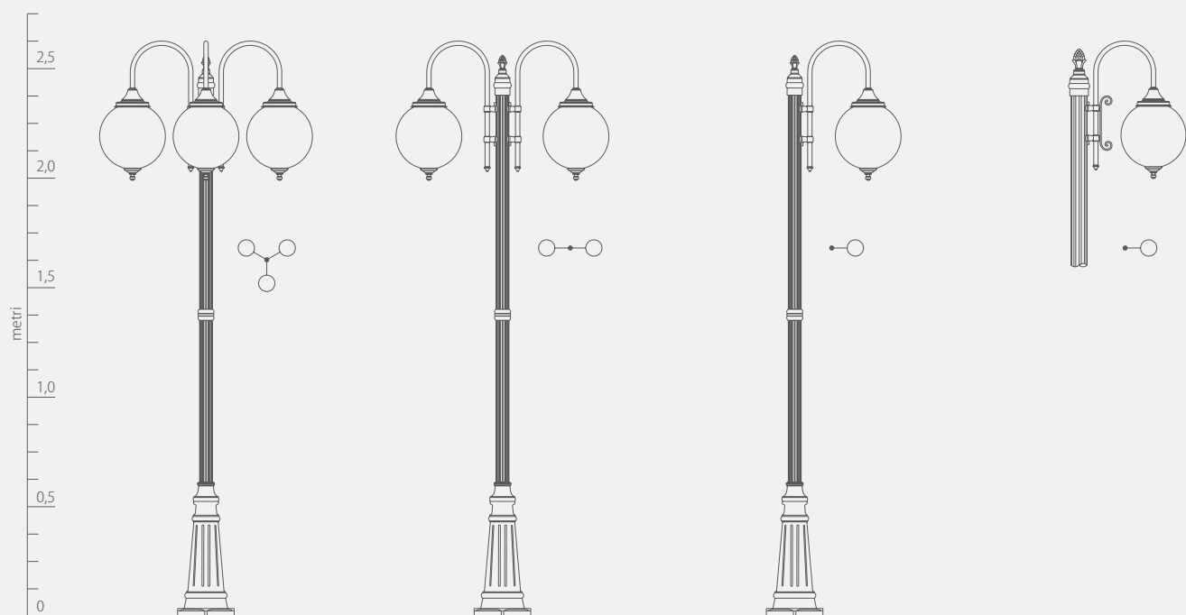
modello: ELIOS 300 articolo: 60.B5/3GP altezza tot. cm 262 palo tipo: 60/B5
