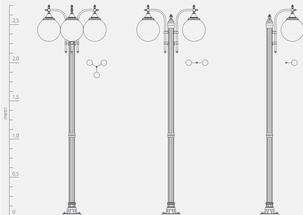
modello: ELIOS 300 articolo: 75/3.90 altezza tot. cm 260 palo tipo: 60
