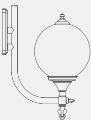
modello: ELIOS 300 articolo: 33A.P misure mm: L480 x H640
