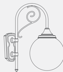
modello: ELIOS 300 articolo: SR.B misure mm: L490 x H600
