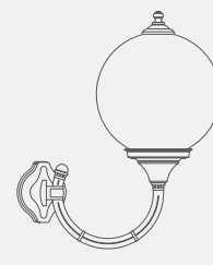
modello: ELIOS 300 articolo: 15A.P misure mm: L460 x H475
