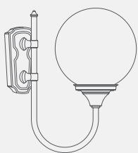
modello: ELIOS 300 articolo: 1A misure mm: L455 x H535
