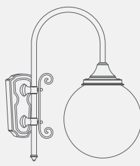
modello: ELIOS 300 articolo: 1GR.B misure mm: L490 x H600
