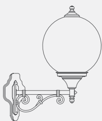
modello: ELIOS 300 articolo: K4B.P misure mm: L480 x H580
