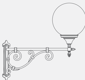
modello: ELIOS 300 articolo: F1.A misure mm: L730 x H700
