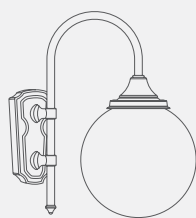
modello: ELIOS 300 articolo: 1B misure mm: L455 x H535
