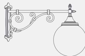
modello: ELIOS 300 articolo: F2.B misure mm: L730 x H700
